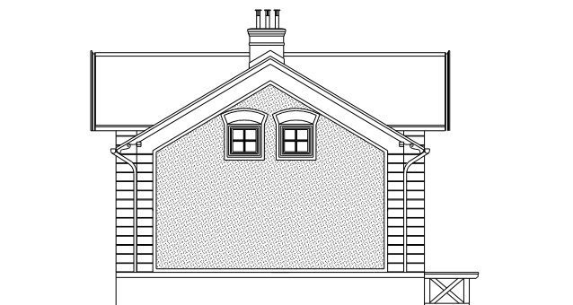
OLDALHOMLOKZAT
